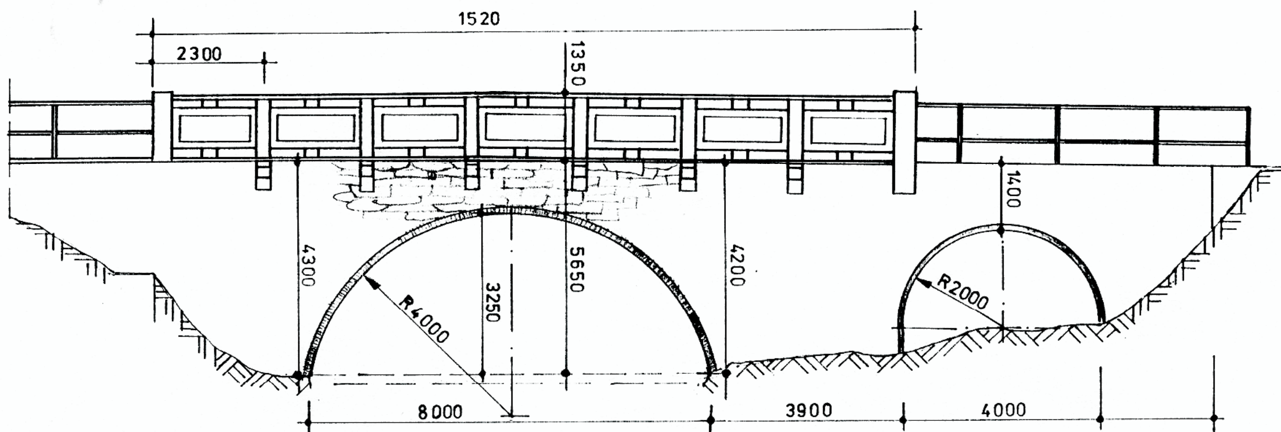
Ansicht Flußaufwärts
