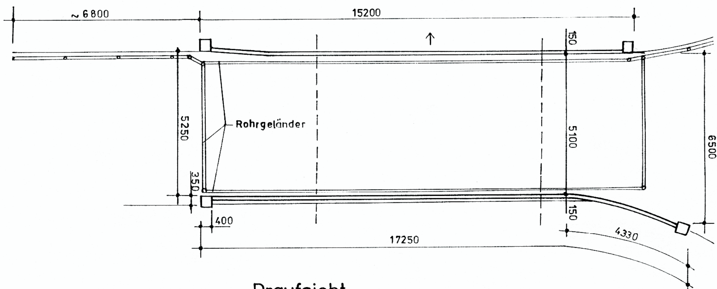
Draufsicht
