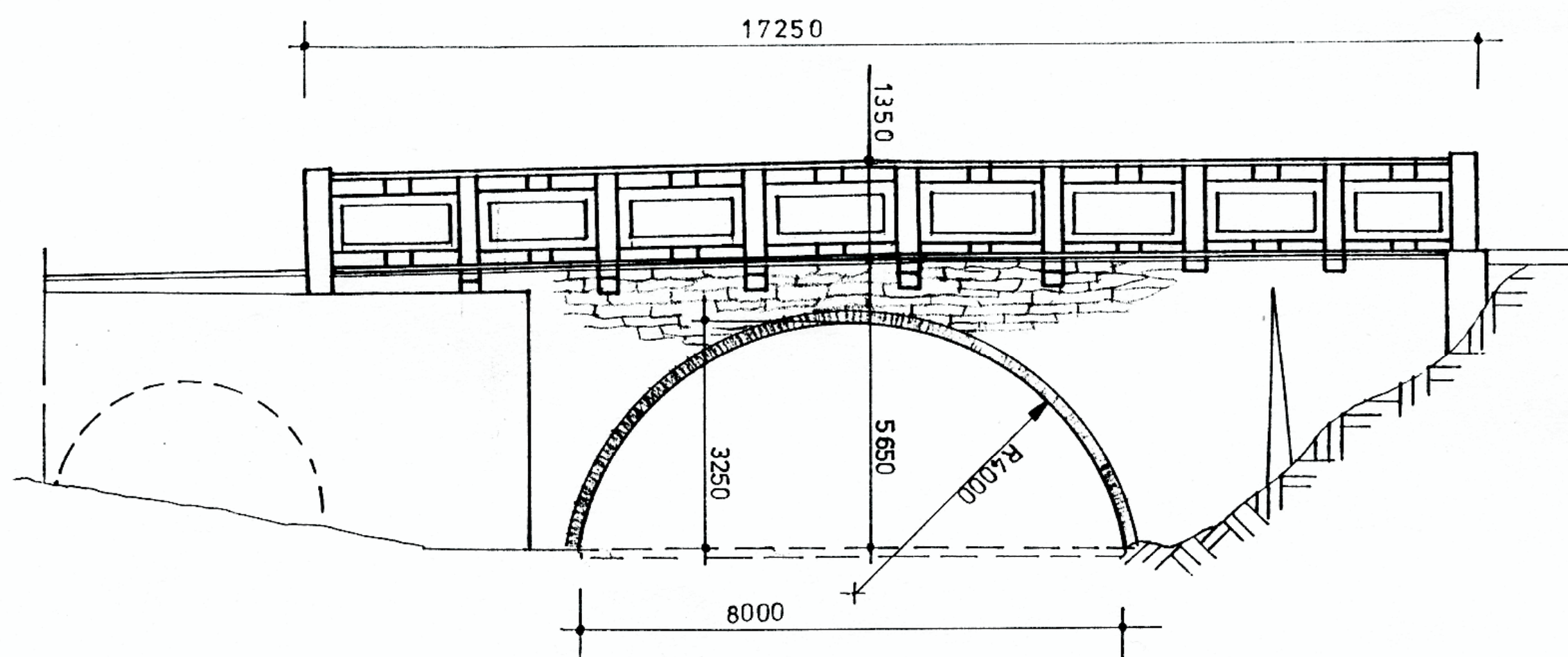
Ansicht Flußabwärts
